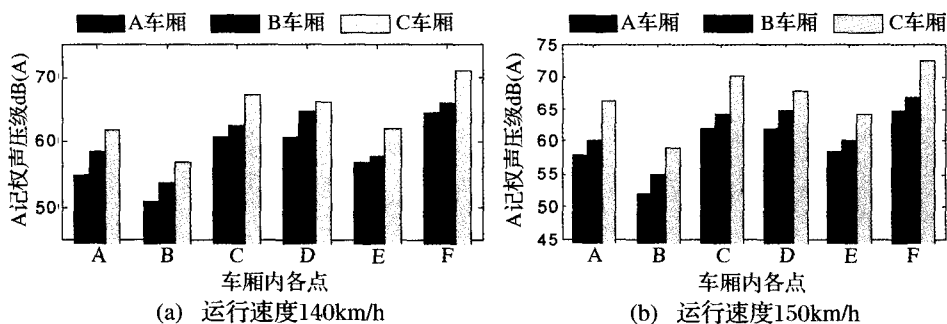
图5 两种车速下三节车厢各测点的A记权声压级
