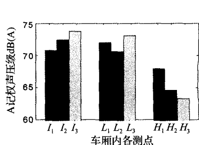
图6 运行速度150km/h时A车厢9 # 包间各测点A计权声压级
